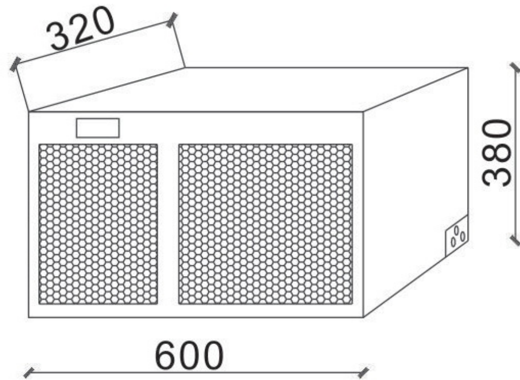
WKSL4000分体机酒窖空调室内机
