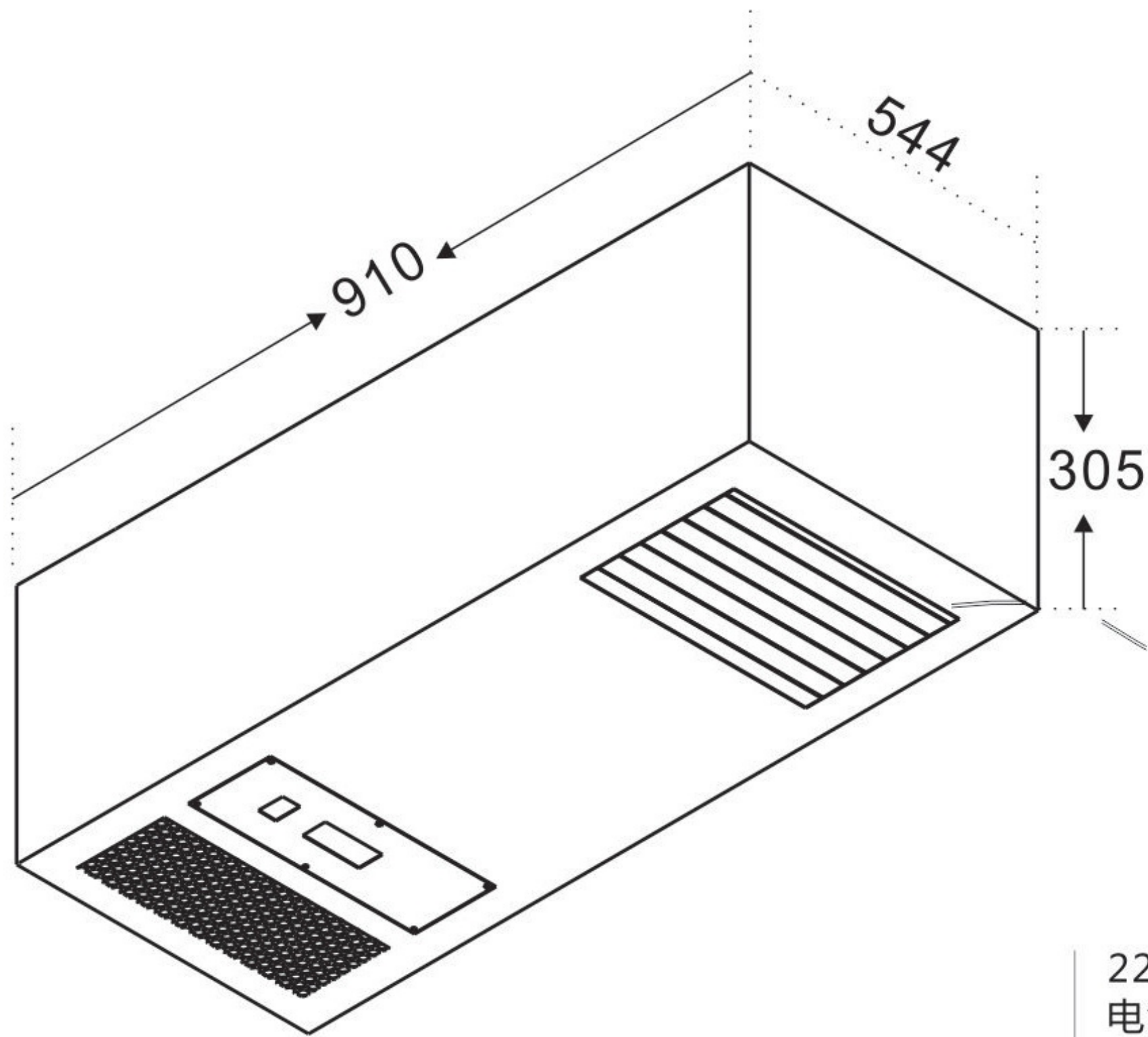
WKSL4000天花机酒窖空调室内机
