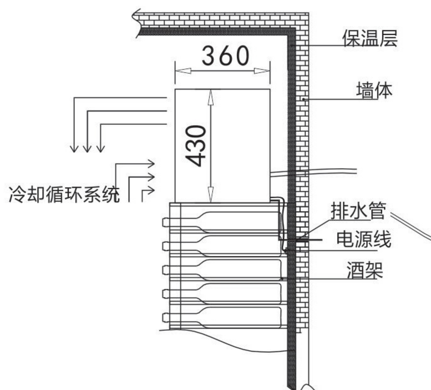
安装剖面图
